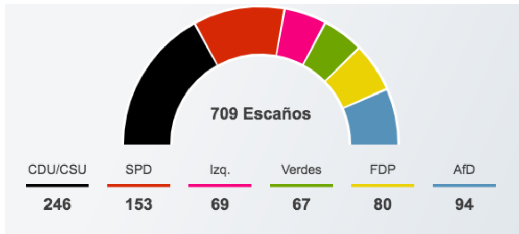
Gráfica 1. Número de escaños para el Bundestag
